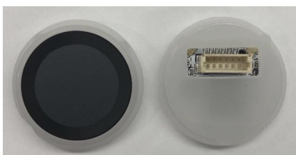
图 1 ML-FPM093D-XX 模组模组
