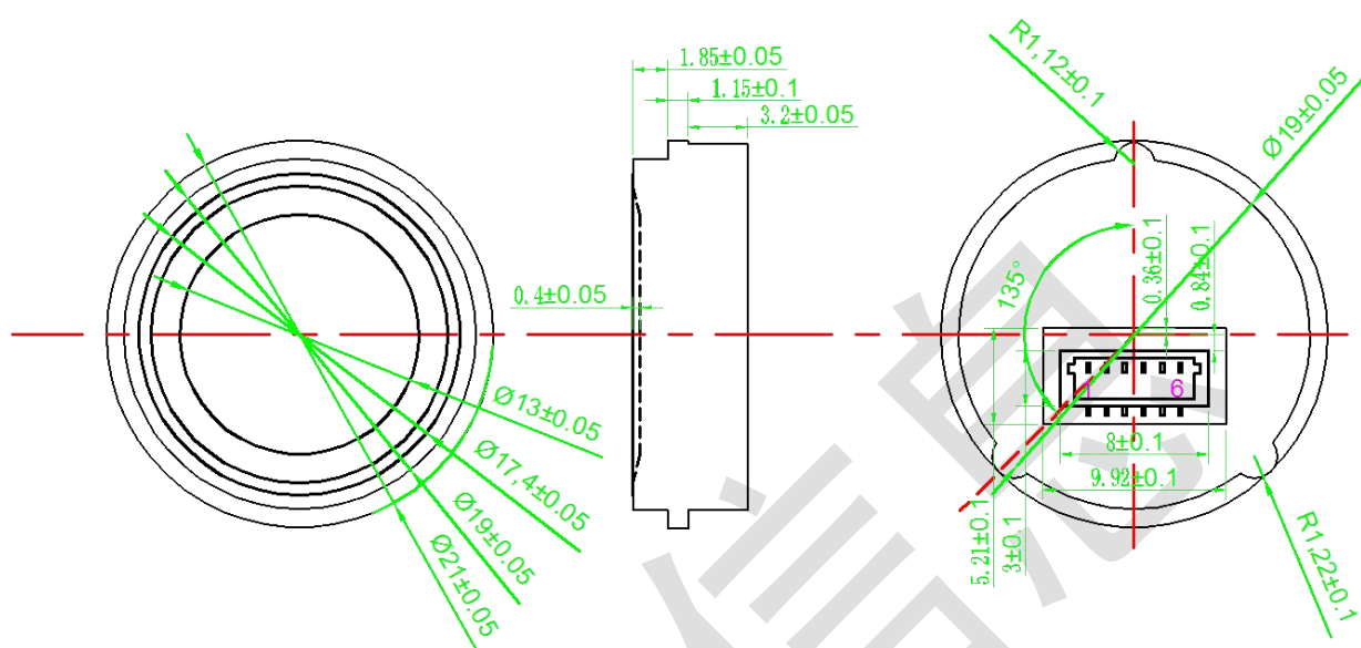
图2 模组结构尺寸
