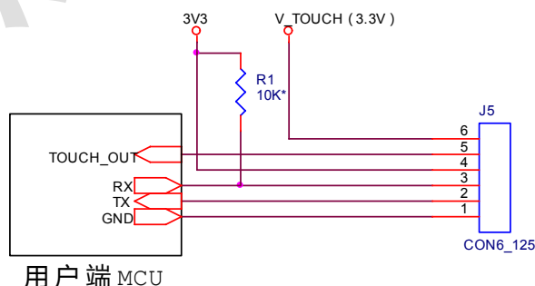
图 6 串口电路设计
